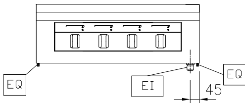
Front aanzicht
